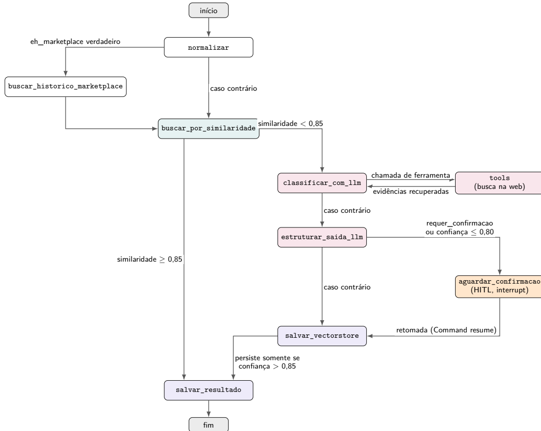
Figura 2 – Grafo de estados do agente de classificação (StateGraph no LangGraph), com a condição de roteamento de cada aresta, conforme codificado na função build_graph .
