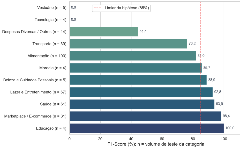
Figura 8 – F1 por categoria de despesa do TF-IDF + Random Forest, melhor modelo do teste cego.
